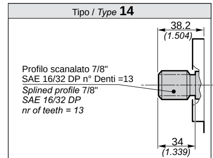
Coppia 240 Nm / Torque 177 ft-lbs
